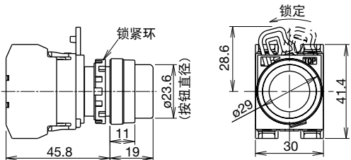
凸头形
