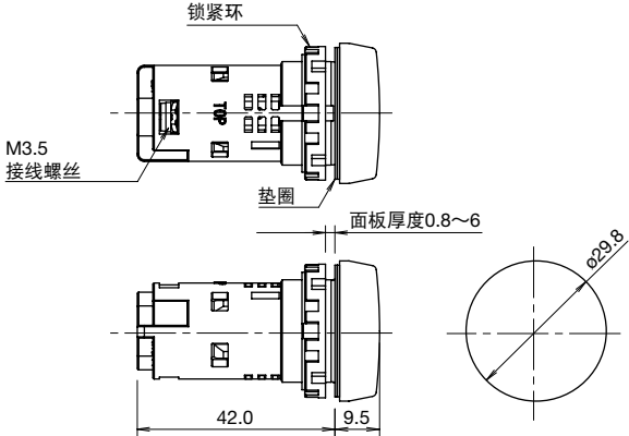
平头形
