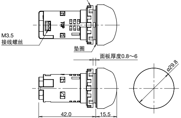
圆凸形
