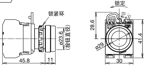
蘑菇头形
