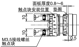
平头形
