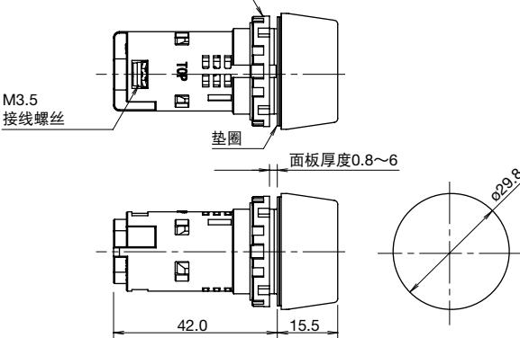
凸头形
