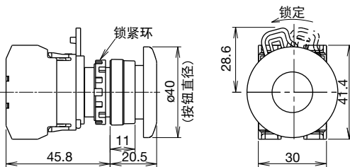
蘑菇头形
